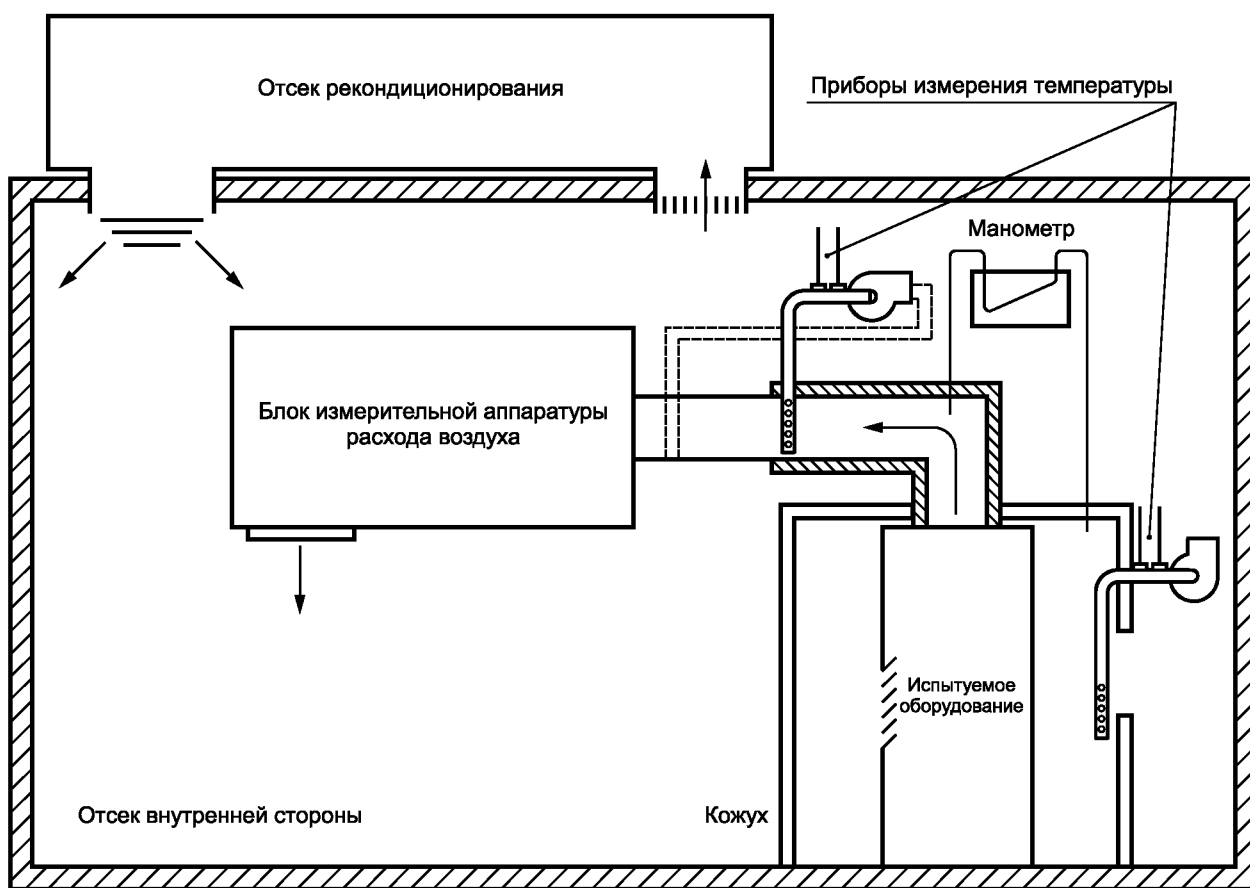
Рисунок F.3 — Компонировка оборудования испытательной камеры для проведения испытаний с использованием кожуха
